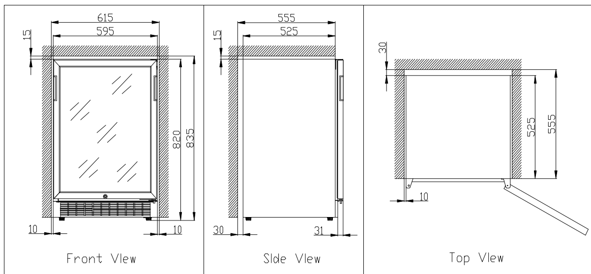
Вид спереди
